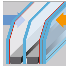
Verbundsicherheitsglas VSG 6 mm einseitig außen mit 3-fach Wärmeschutz- verglasung , Ug 0.7
