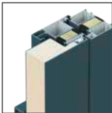
einseitig flügelüberdeckend (48 mm)
