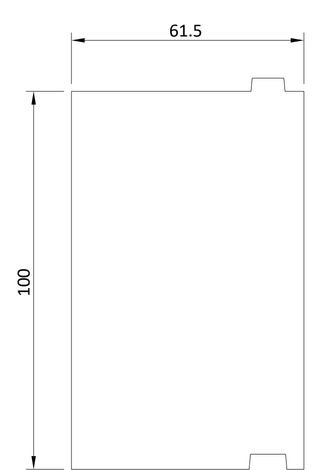
83303 Unterbauprofil Base profile
