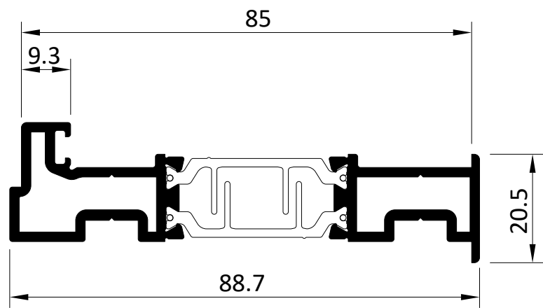
91575 Kopplung Coupling
