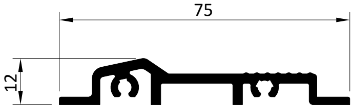
2733 Schwelle Threshold
