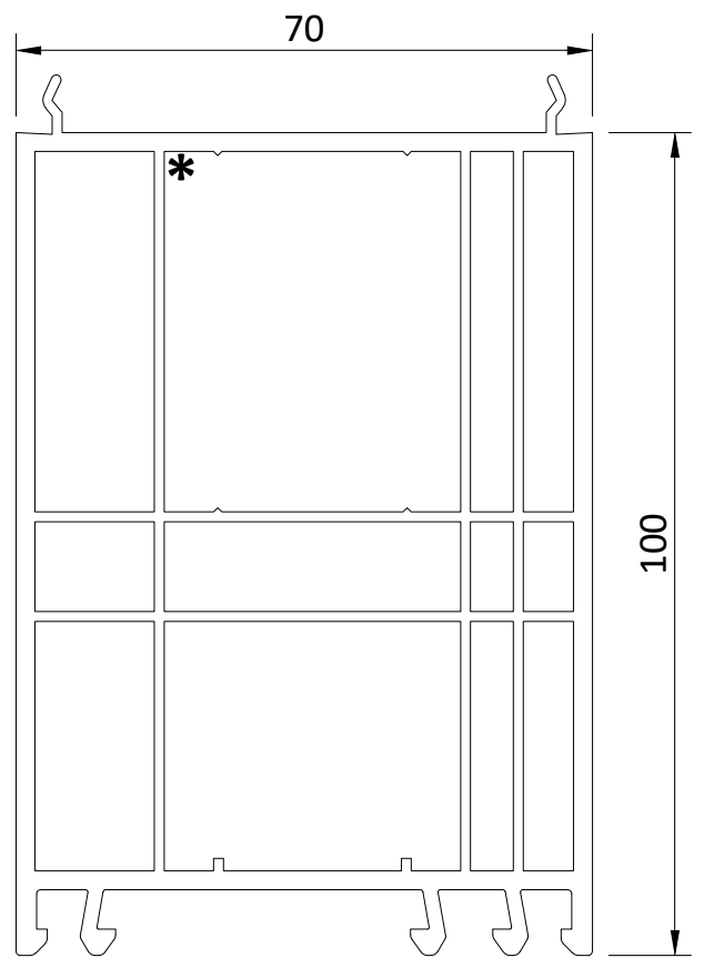
83154 Aufdopplung Doubling → 83150
