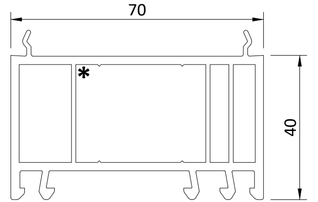
83152 Aufdopplung Doubling → 83150
