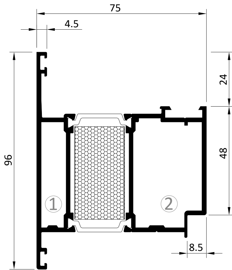
1428/1448/14027 Flügel Leaf Isolator Insulation 2213
