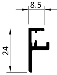
2732 Abschlussprofil Cover profile
