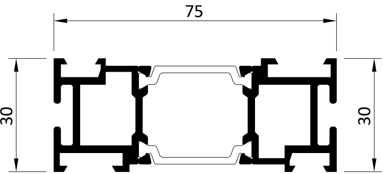
1402 Basisprofil Base profile
