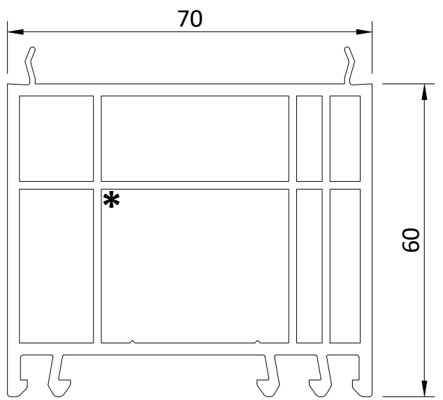
83153 Aufdopplung Doubling → 83150
