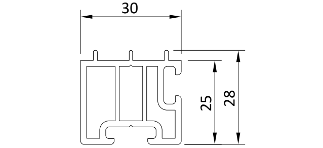
83155 Basisprofil Base profile
