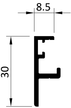
2731 Abschlussprofil Cover profile → Panikflügel Panic leaf
