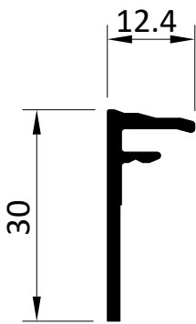
2784 Klipsprofil Clip profile
