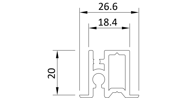
8315 Türabschluss Door ending → 1434
