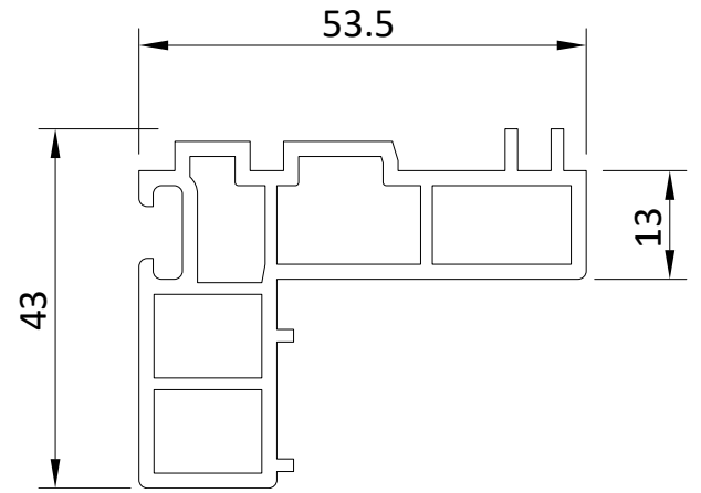
8333 Basisprofil Base profile
