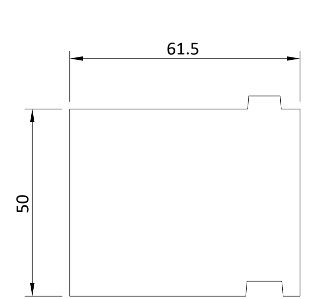
83302 Unterbauprofil Base profile
