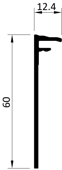
2785 Klipsprofil Clip profile
