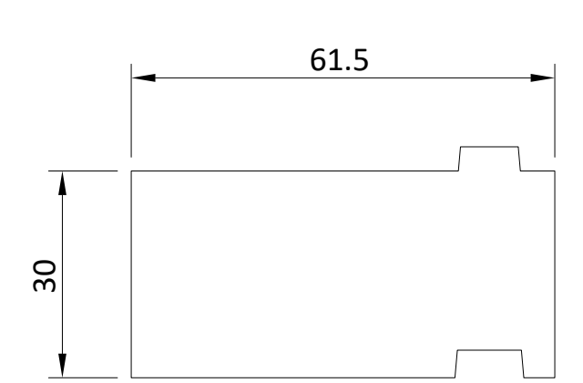
83301 Unterbauprofil Base profile
