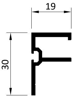
4814 Anschluss Connection
