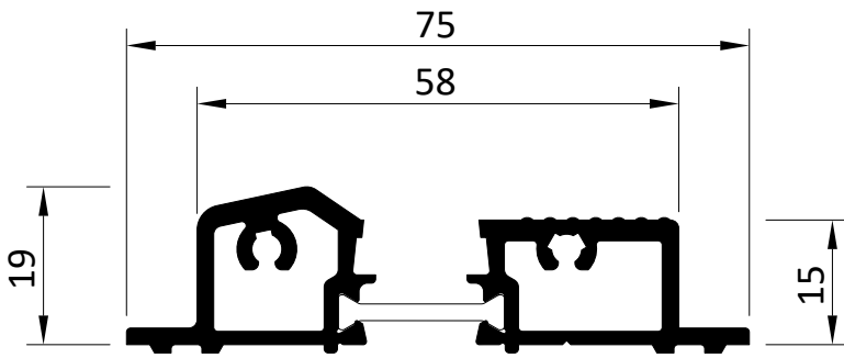
1404 Schwelle Threshold
