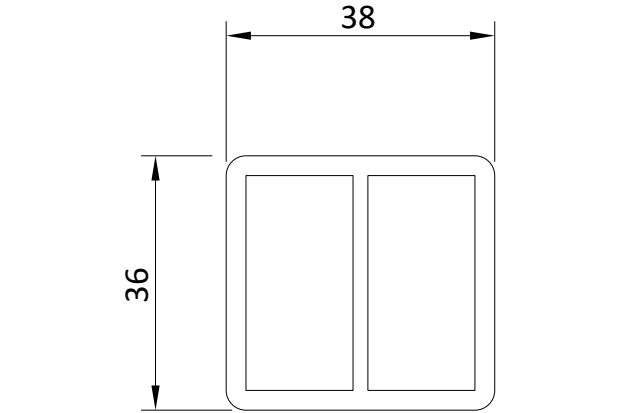
8334 Rohr Pipe 38 x 36 mm
