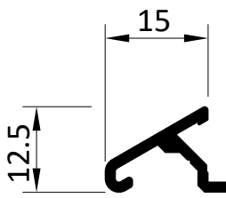
1460 Wetterschenkel Rain guard
