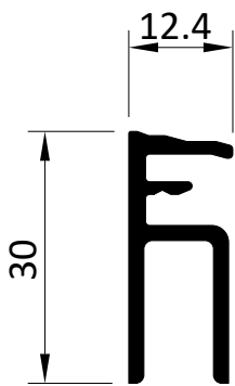
2788 Klipsprofil Clip profile
