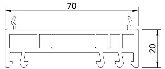
83151 Aufdopplung Doubling → 83150
