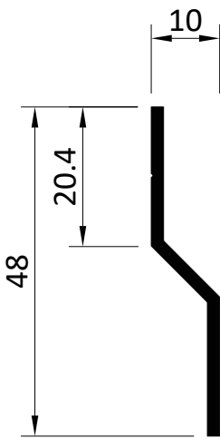
27111 Regenabweiser Rain deflector
