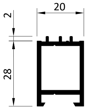
2755 Verbreiterungsprofil Extension profile
