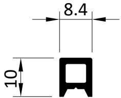
27145 Zusatzprofil Additional profile → Türflügel Door leaf
