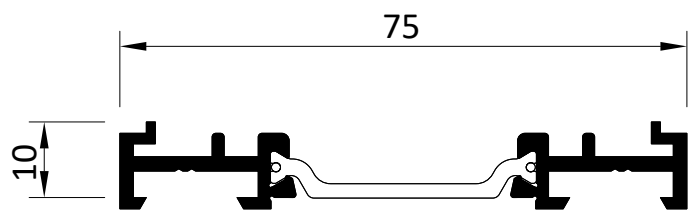
14101 Ausgleichprofil Adjustment profile
