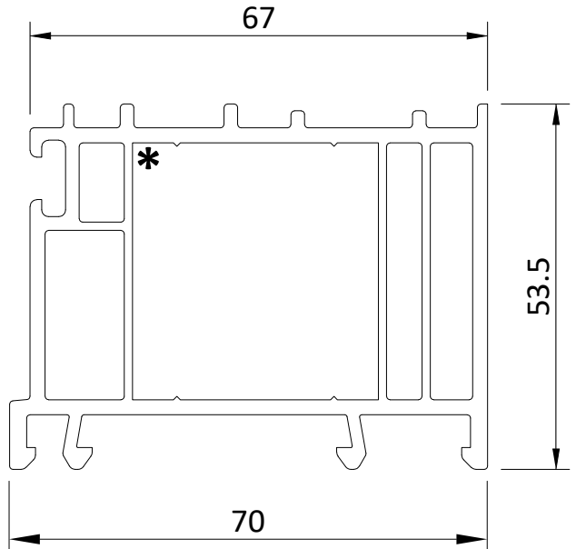
83150 Basisprofil Base profile
