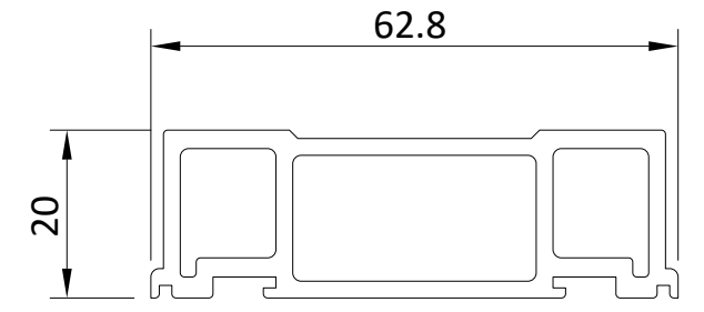
8311 Türabschluss Door ending → 1434
